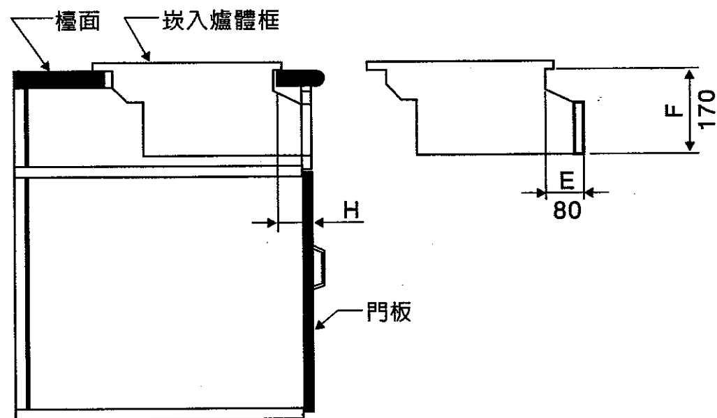
嵌入爐安裝檯面挖孔尺寸說明圖
